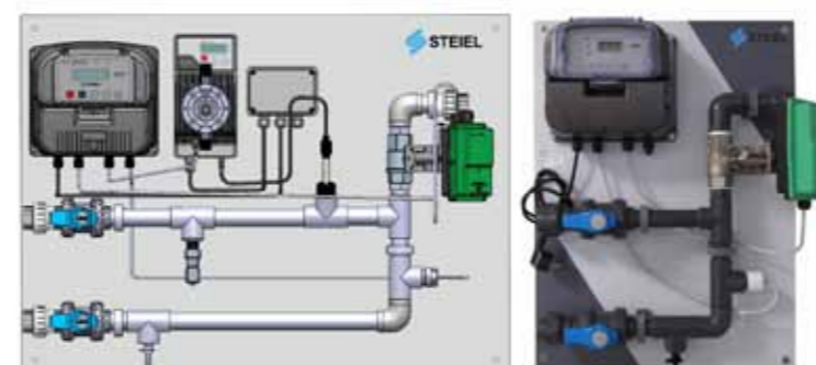
Sistemas de purga automática para torres de enfriamiento, con recuperación de agua. Panel con bomba y medición ORP / Panel sin bomba.
